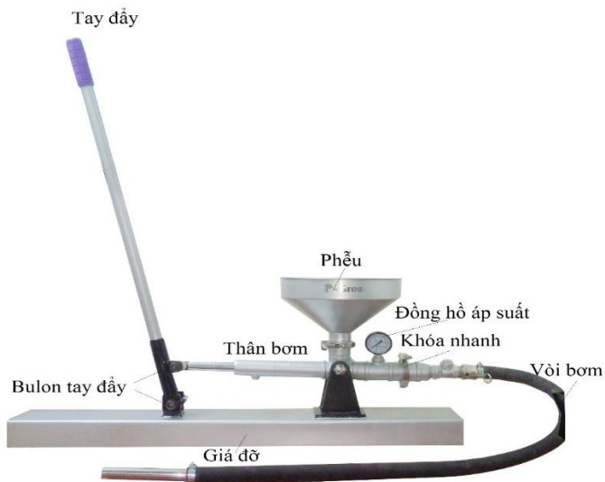
Sơ đồ lắp đặt máy bơm vữa
